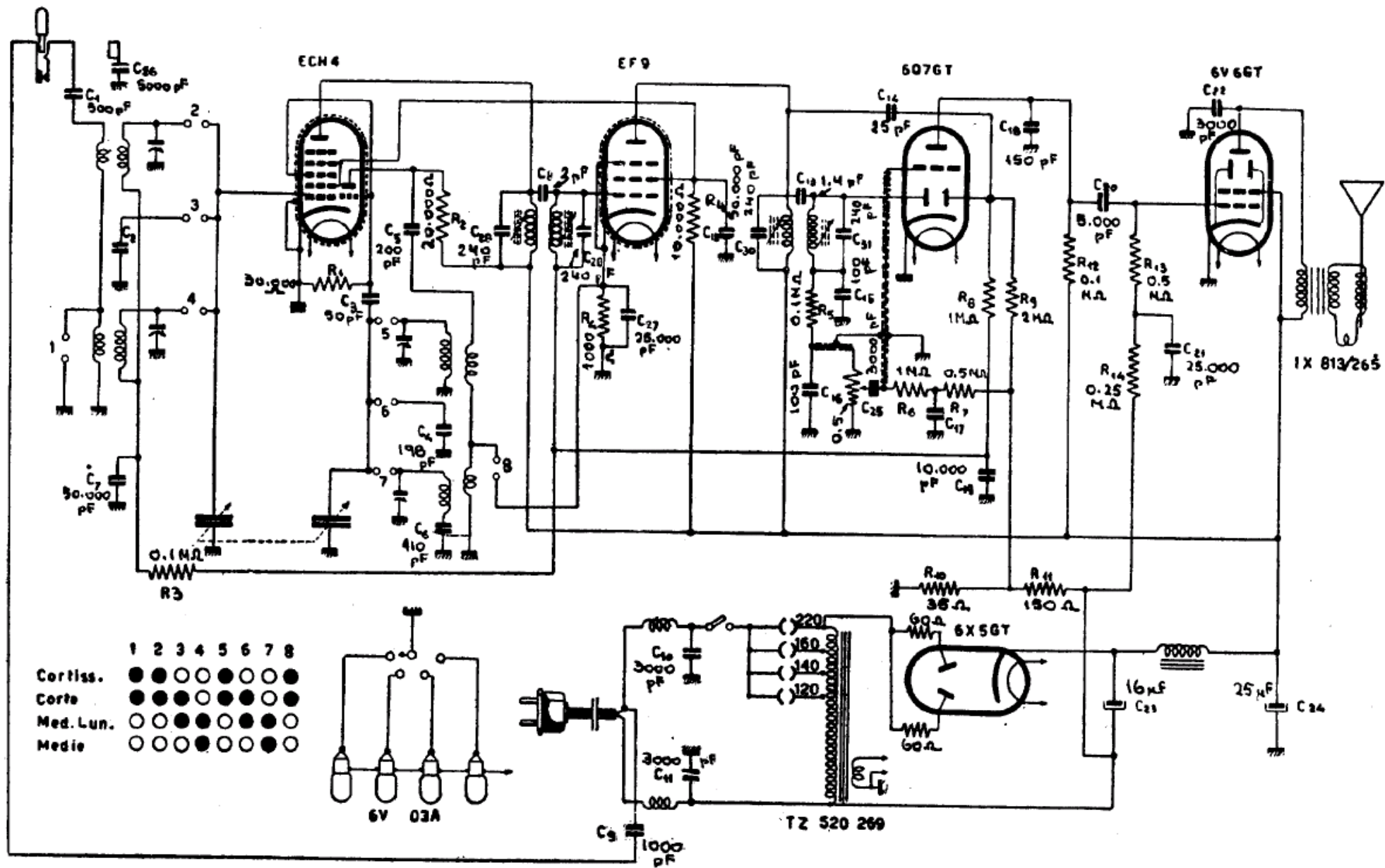
PHONOLA RADIO - Mod. 573 - Supereterodina con gamma onde medie suddivisa. Potenza circa 1,5 watt. Media frequenza: 470 kc/s. Produzione 1945-46.
